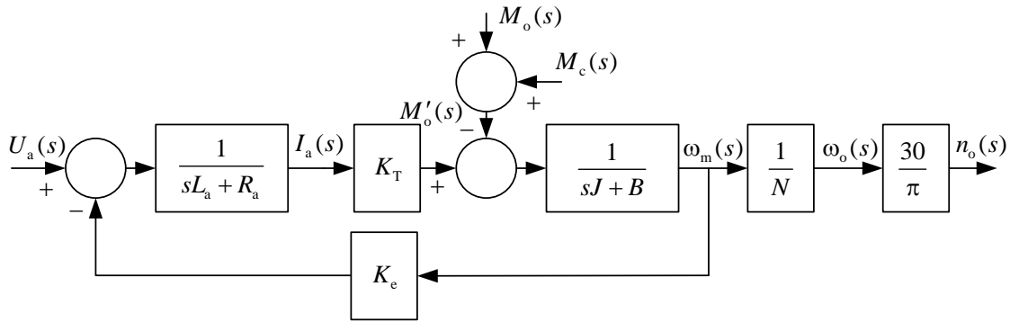
Сл. 3.15 Блок дијаграм мотора управљаног напонам индукта са утицајем Coulomb-овог трења
