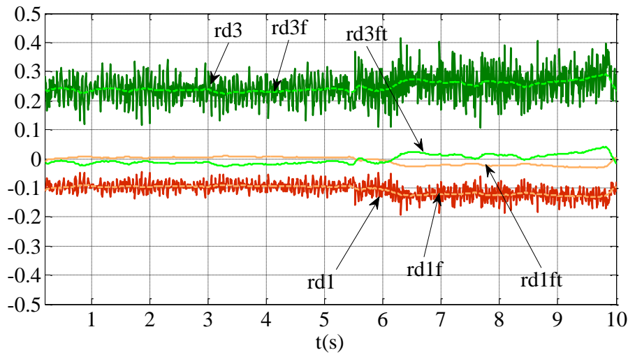
Сл. 4.65 Прва и трећа координата дирекционог вектора у одзиву на отказ -\Delta M_0 .
