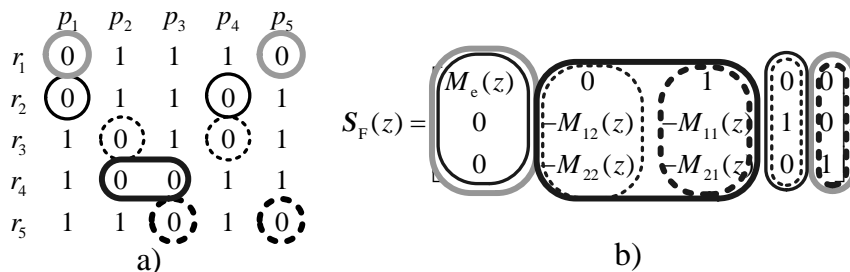
Сл. 4.8 а) Скоро потпуна, хомогена спецификација одзива; б) одговарајуће S_i(z) матрице
