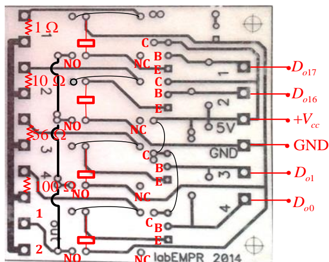
Сл. 3.6 Плочица са релејима за промену отпорности R_1
