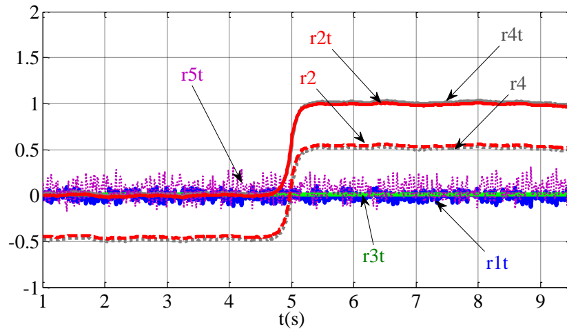
Сл. 4.53 Филтрирани и транслирани рачунски резидуали при отказу \Delta n_0 у 5s
