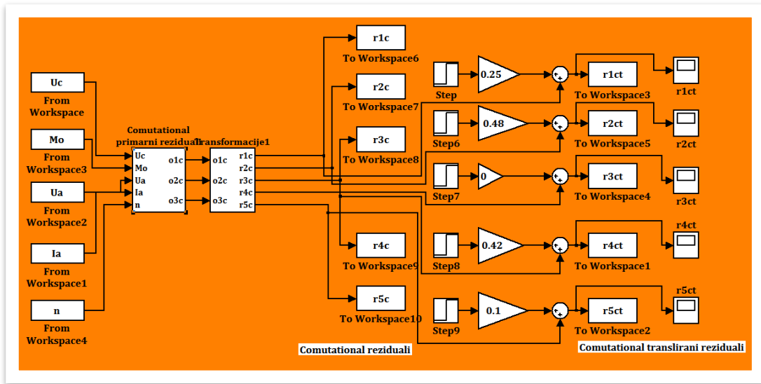
Сл. 4.48 Simulink модел транслираних резидуала код структурне матрице формирање на основу модела система
