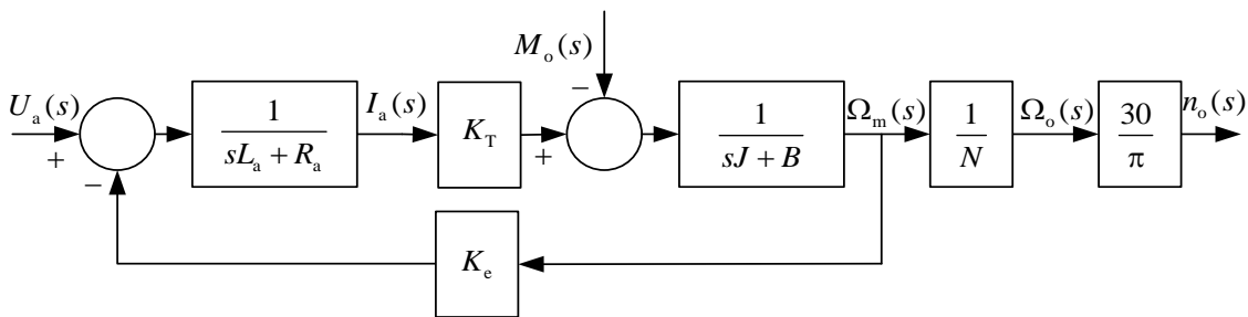
Сл. 3.16 Блок дијаграм мотора управљаног напонам индукта
