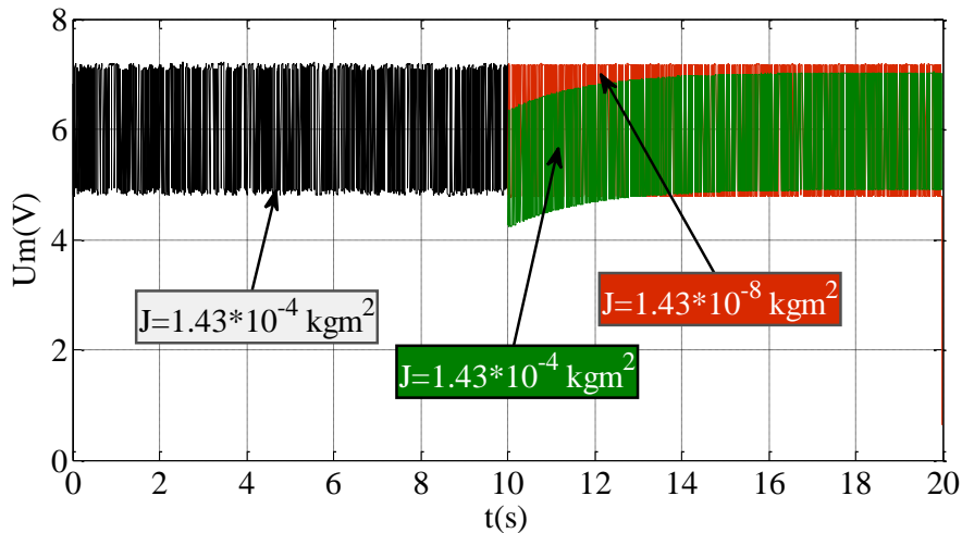
Сл. 5.17 Излазни напон појачавача при промени J у 10s
