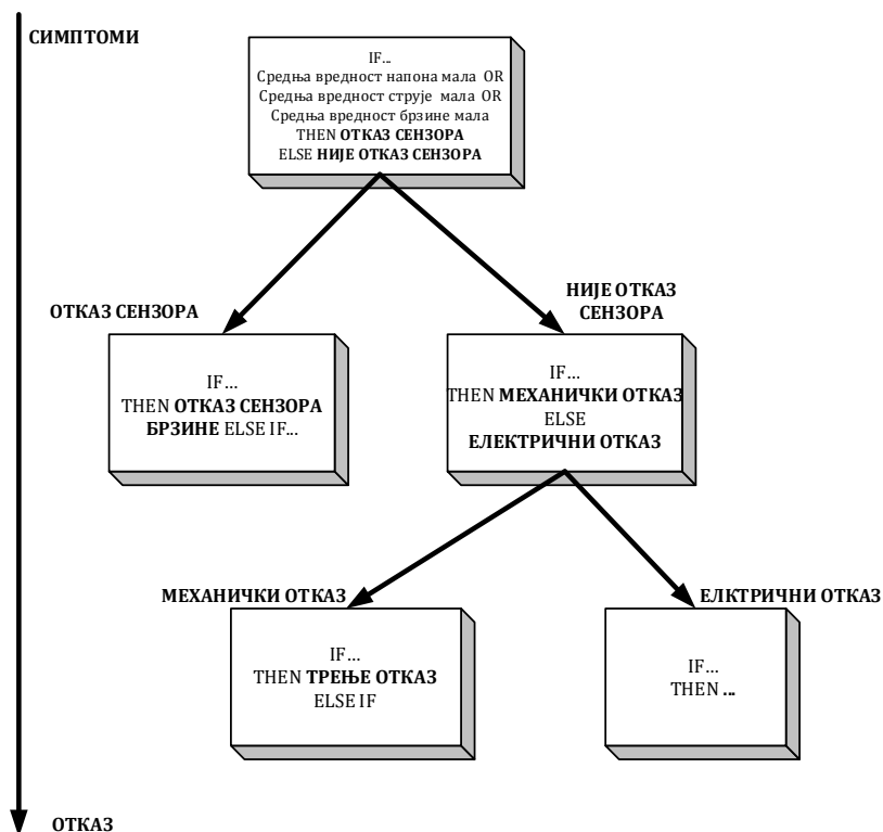
Сл. 2.1 Хијерархијски алгоритам одлучивања.
