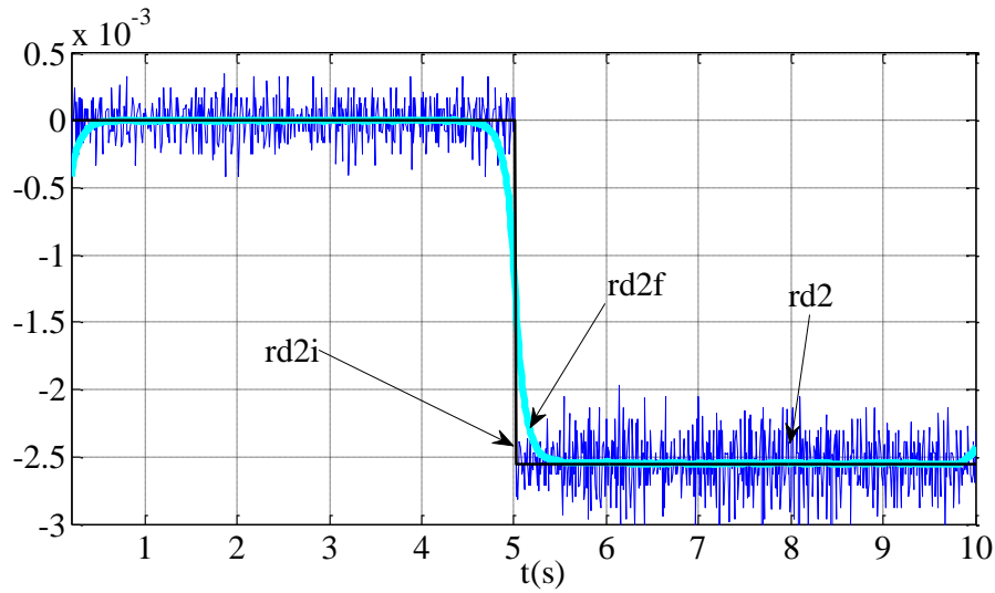
Сл. 4.64 Друга координата дирекционог вектора у одзиву на отказ -\Delta M_0 .
