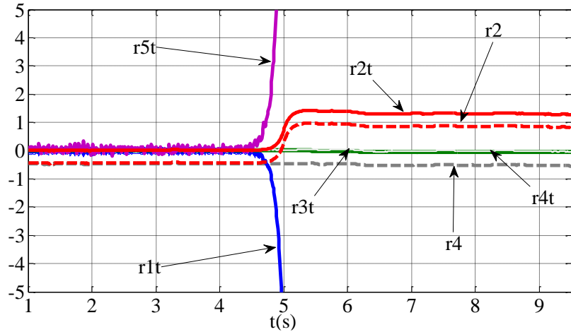
Сл. 4.50 Филтрирани и транслирани рачунски резидуали при отказу -\Delta M_0 у 5s
