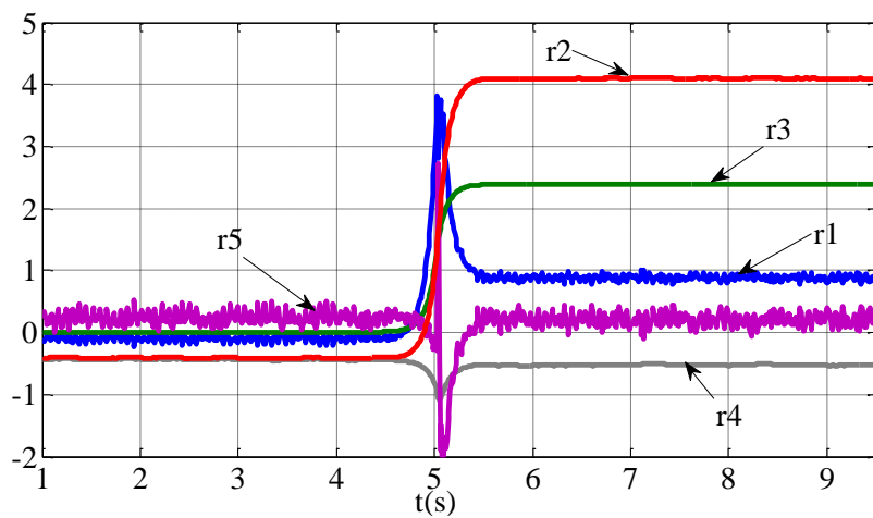
Сл. 4.15 Филтрирани рачунски резидуали при отказу \Delta U_c у 5s
