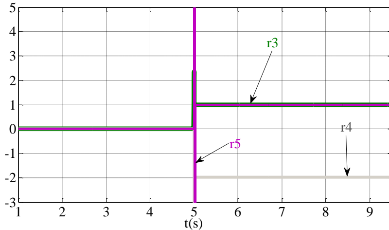
Сл. 4.20 Интерни резидуали при отказу \Delta U_a у 5s
