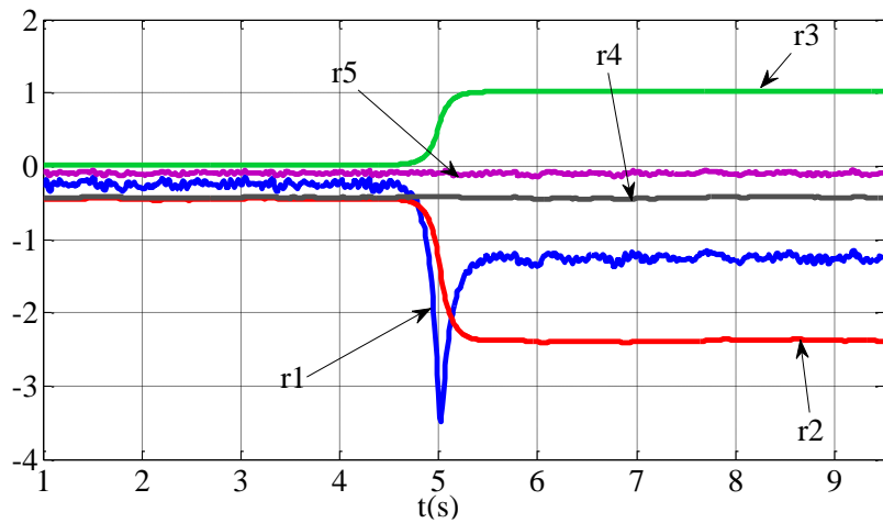
Сл. 4.39 Рачунски филтрирани резидуали при отказу \Delta U_a у 5s
