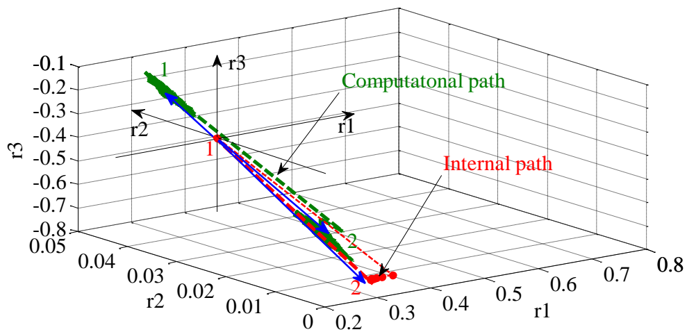
Сл. 4.69 Рачунске и интерне путање при \Delta I_a
