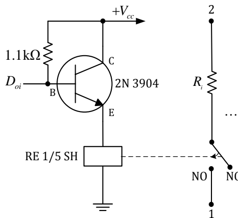
Сл. 3.5 Електронска шема основног дела релејне плочице
