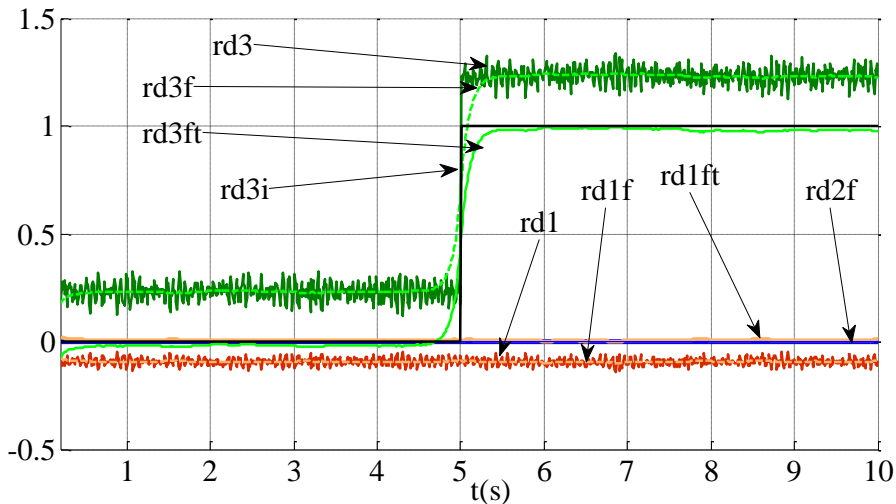
Сл. 4.68 Координате дирекционог вектора у одзиву на отказ \Delta U_a
