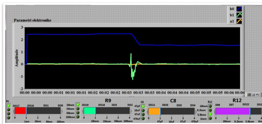
Сл. 5.6 Део Front Panela LabVIEW на коме су приказани процењени параметри појачавача применот Алгоритма клизног интеграла
