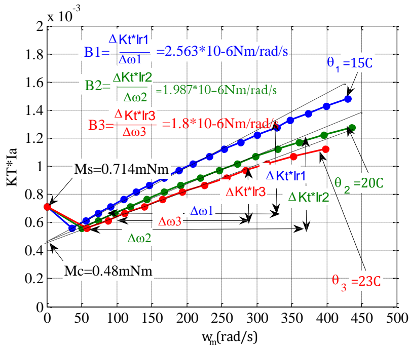
Сл. 3.13 Експериментално одређивање трења у мотору једносмерне струје при температурама околине: \theta_1 = 15^\circ \text{C} , \theta_2 = 20^\circ \text{C} , \theta_3 = 23^\circ \text{C}
