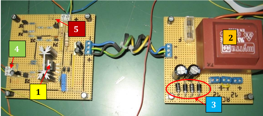
Сл. 3.2 Линеарни електронски појачавач (1) операциони појачавач TDA2030(A), (2) трансформатор; (3) диодни исправљач; (4) улаз – управљачки напон U_c(t) (5) излаз – референтни напон индукта мотора U_m(t) † тј. струја индукта I_a(t) ;
