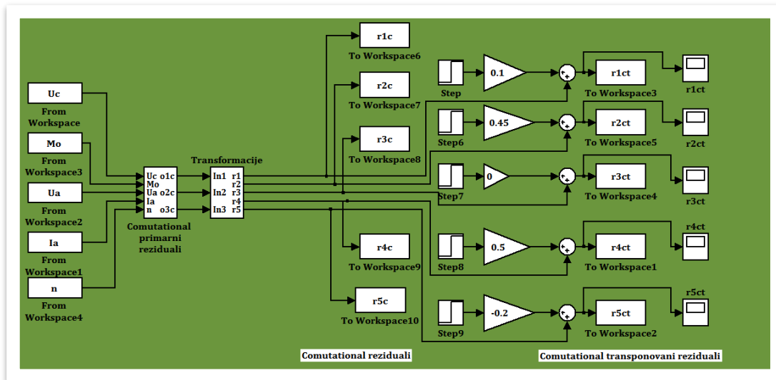
Сл. 4.47 Simulink модел транслираних резидуала код структурне матрице формиране на основу модела система
