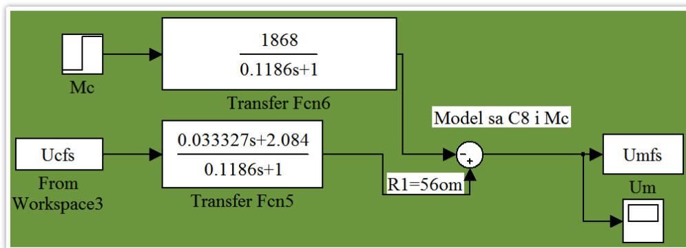
Сл. 5.26 Симулациони модел појачавача при отказу R_1 = 56 \Omega
