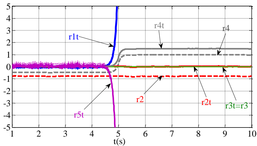
Sl.7.1. Сл. 4.52 Филтрирани и транслирани рачунски резидуали при отказу \Delta I_a у 5s увећани приказ
