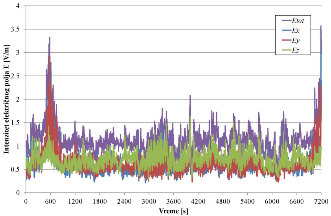
Slika A.17 Intenzitet električnog polja u zavisnosti od vremena za scenario 6
