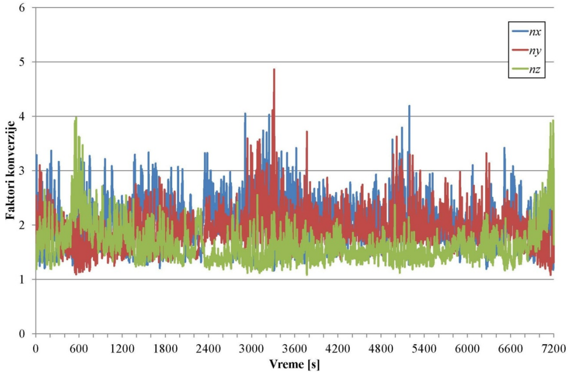
Slika A.18 Faktori konverzije n_x , n_y i n_z u zavisnosti od vremena za scenario 6
