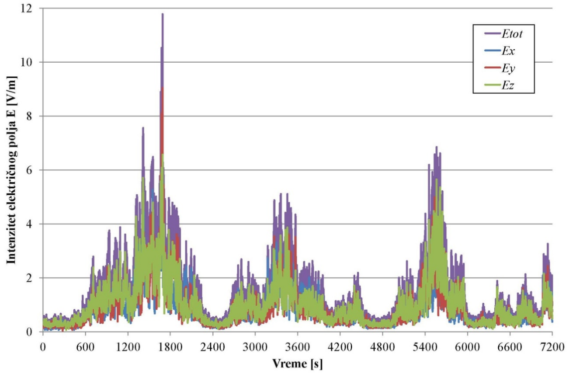
Slika 5.1 Intenzitet električnog polja u zavisnosti od vremena za scenario 1
