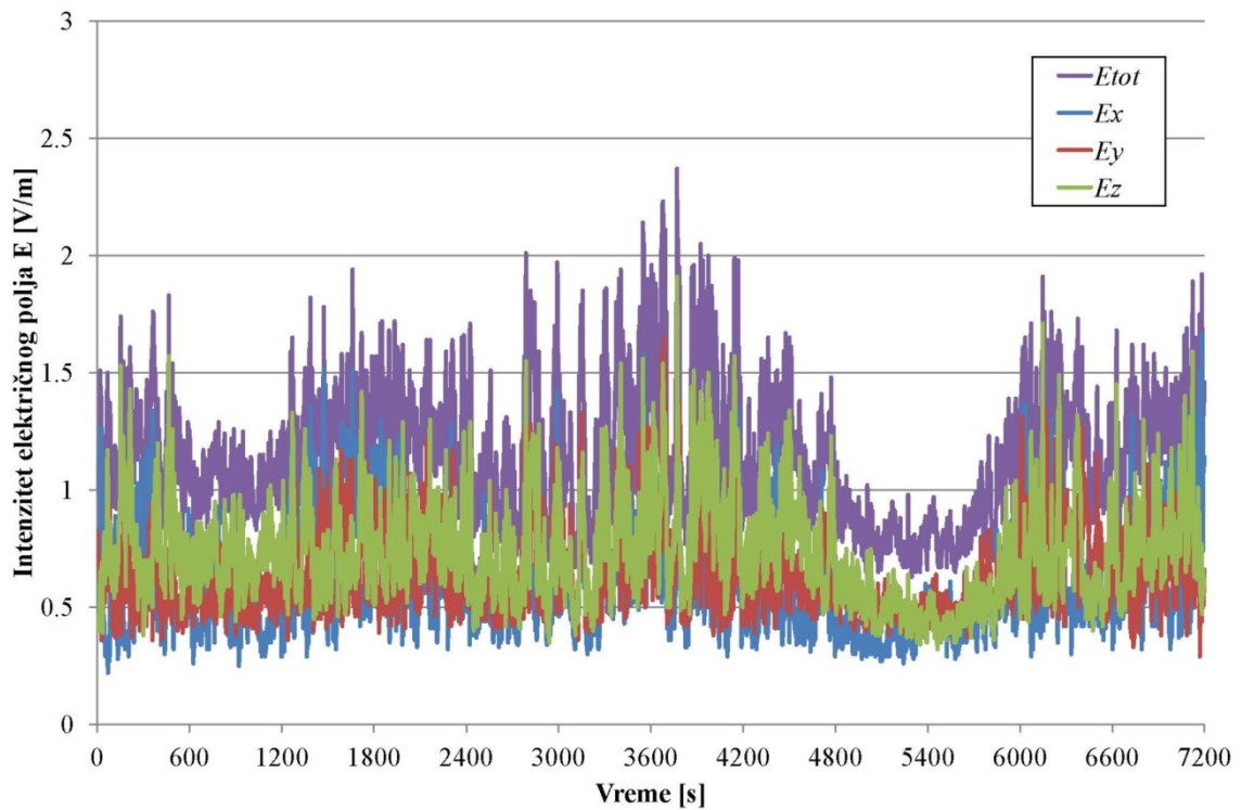
Slika A.5 Intenzitet električnog polja u zavisnosti od vremena za scenario 3
